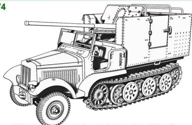
7,62cm FK.36 (R) auf mZgkw 5t "Diana" SdKfz.6/3
